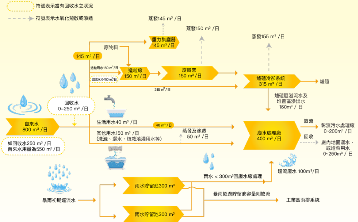
鋼聯用水平衡圖
